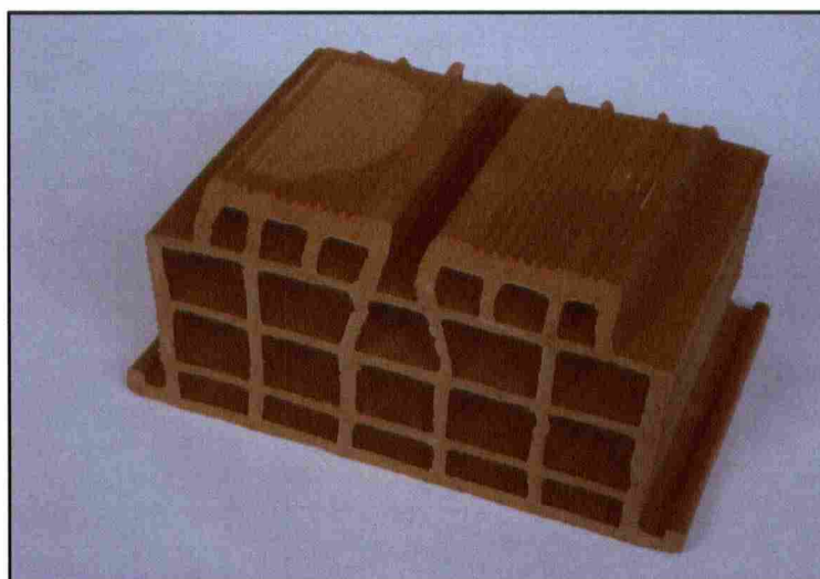
Blocco in laterizio denominato: PANNELLO 20/40 S
