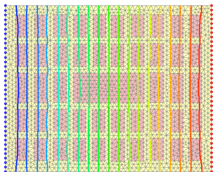
SPESSORE PARETE 25 cm
